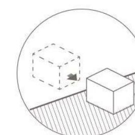
Object Left
